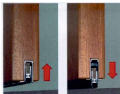
SEUIL MÉCANIQUE SOULEVABLE INTÉGRÉ AU VANTAIL
